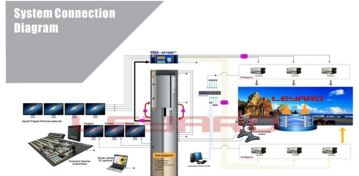
Diagrama de conexión para FORO de TV
